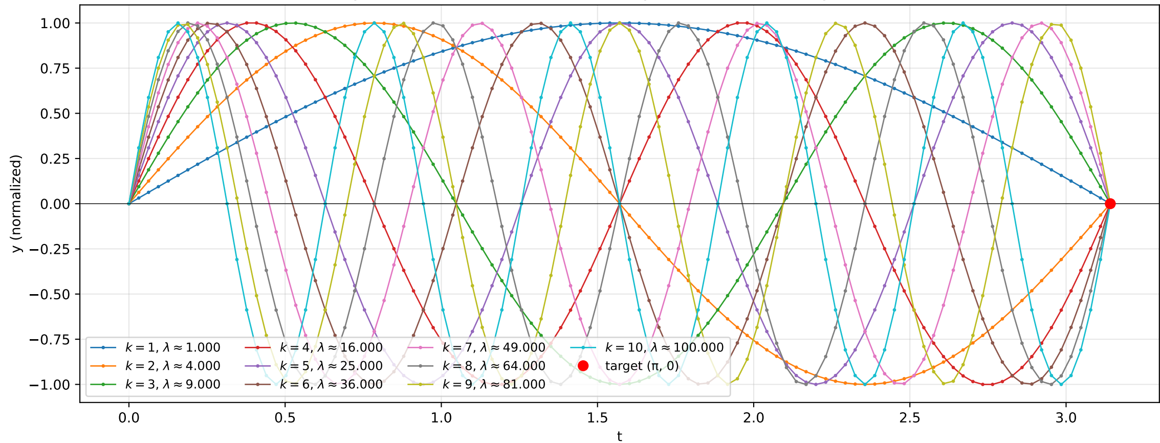
Eigenfunctions via Prüfer on uniform grid (n=100) for 10 eigenvalues
